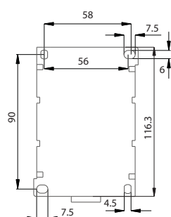
CEM 80CN
