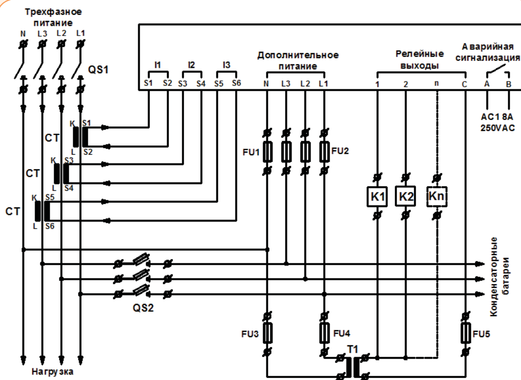
Правильное подключение
