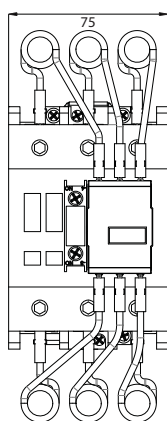
CEM 32... 80CN
