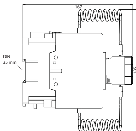
CEM 32... 80CN
